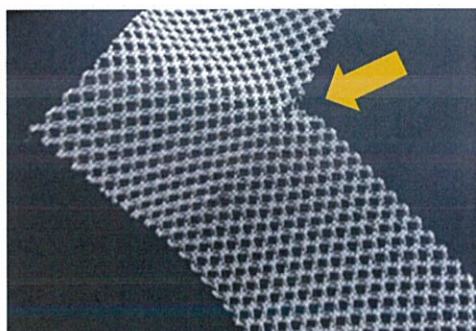
写真2. メッシュ鋭角形状部分の破損状態
